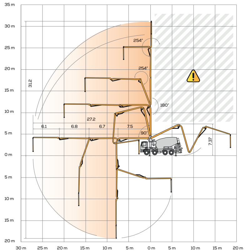
Verteilmast MK32L
